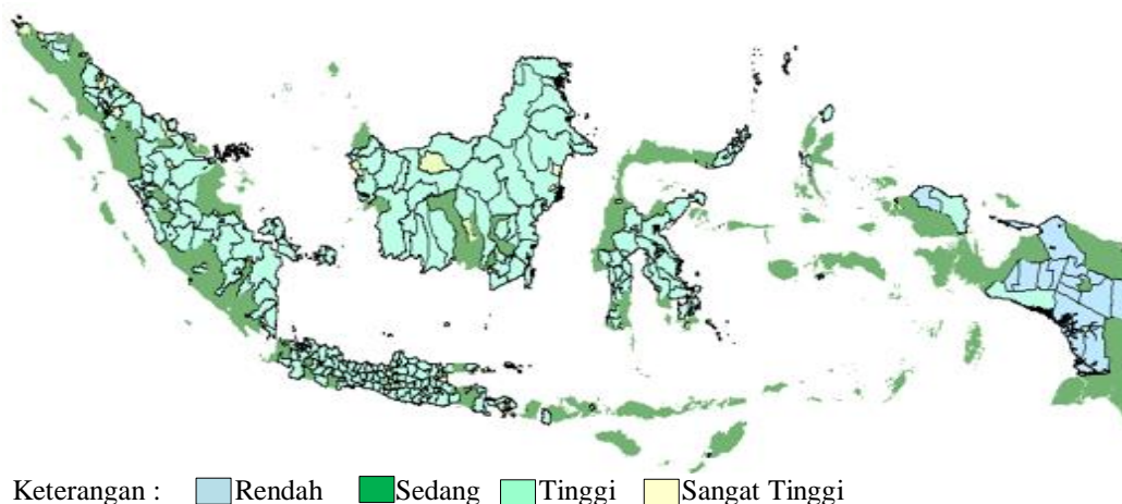
Gambar 3. Sebaran Hasil Kluster Metode Fuzzy C-Means
