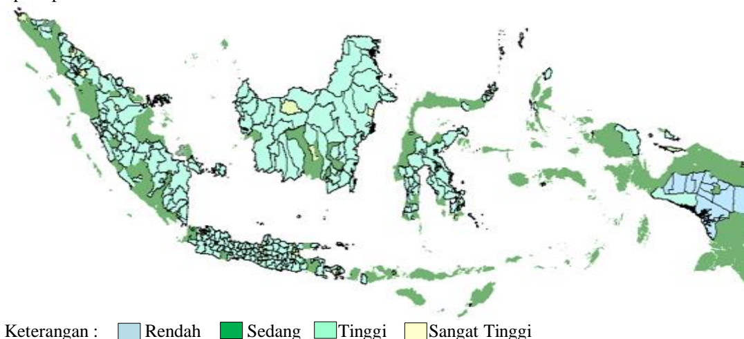
Gambar 2. Sebaran Hasil Kluster Metode K-Means
