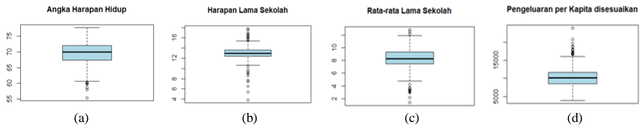
Gambar 1. (a) Boxplot Angka Harapan Hidup Menurut Kabupaten/Kota di Indonesia Tahun 2021, (b) Boxplot Harapan Lama Sekolah Menurut Kabupaten/Kota di Indonesia Tahun 2021, (c) Boxplot Rata-rata Lama Sekolah Menurut Kabupaten/Kota di Indonesia Tahun 2021, (d) Boxplot Pengeluaran per Kapita disesuaikan Menurut Kabupaten/Kota di Indonesia Tahun 2021
